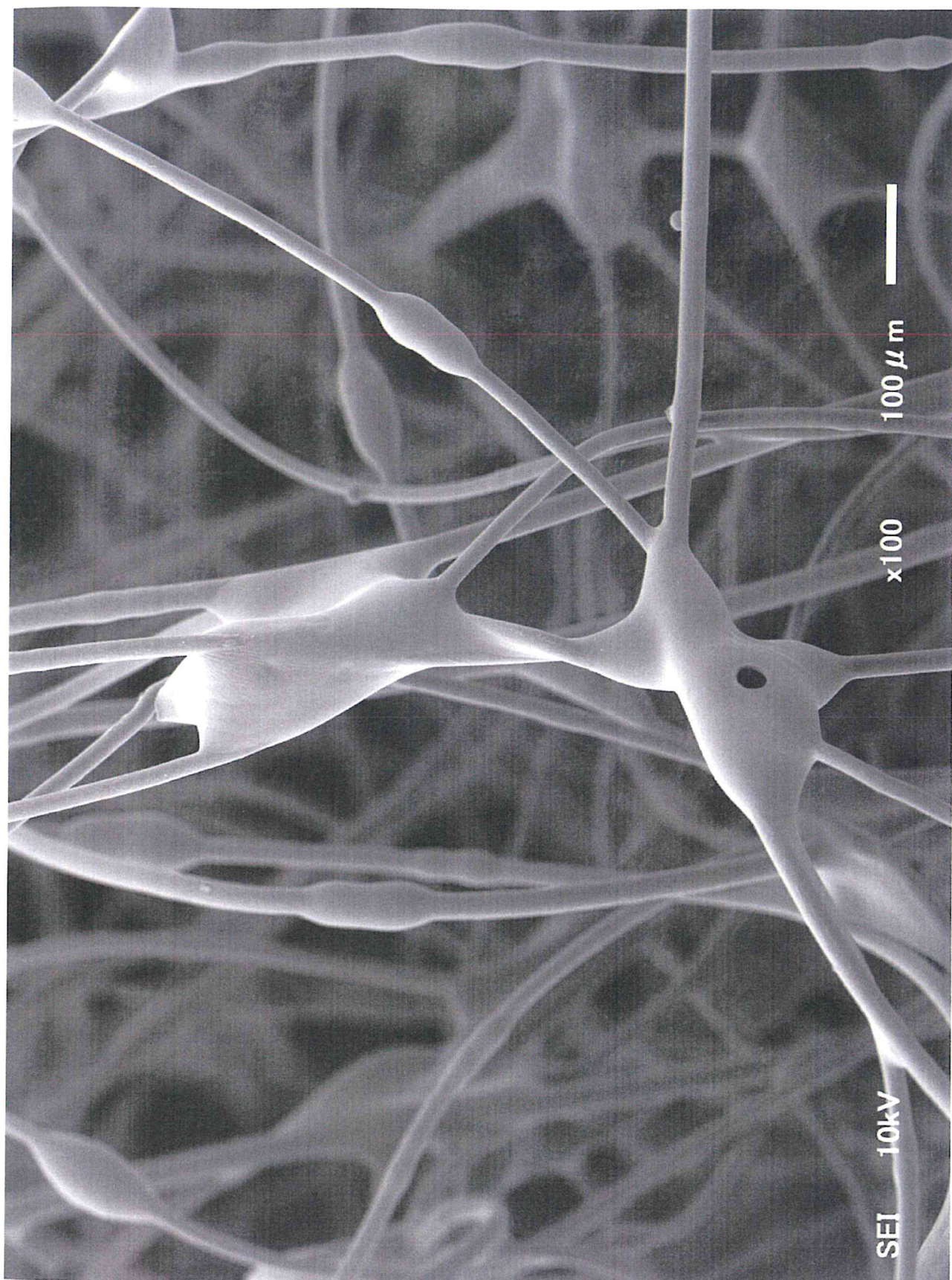
写真8 業務用エアコンATフィルター未使用の走査型電子顕微鏡写真
